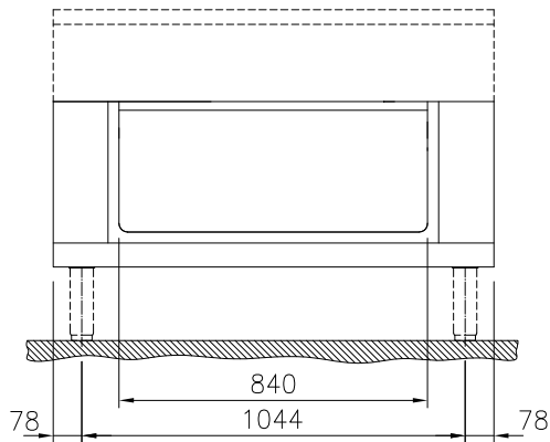
Zij aanzicht
